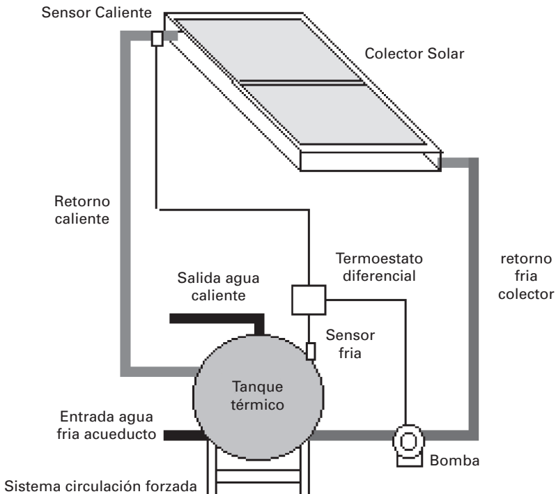
Esquema de instalación de energía solar térmica
