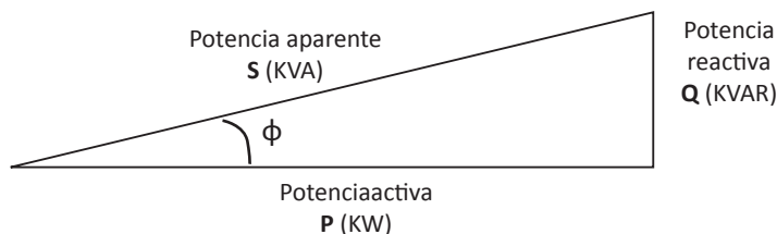
Figura 4. Triángulo de potencias eléctricas
